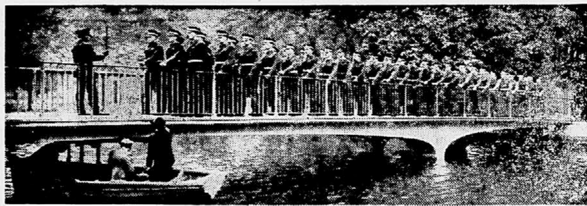
Nedavno zgrajeni most v parku St. James v Londonu so preizkusili pod težo 22 ton korakajočih gardistov. Most je zgrajen iz prednapetega betona. Medtem ko so vojaki korakali čez most dobre ure, so stokovniki v čolnu pod mostom merili tresljaje z instrumenti.
