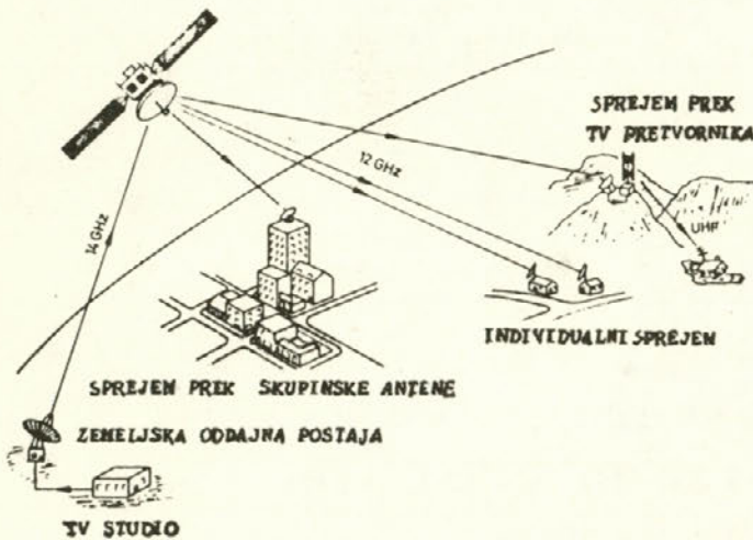
SKICA 4 - Sprejemanje signalov prek TV satelita
