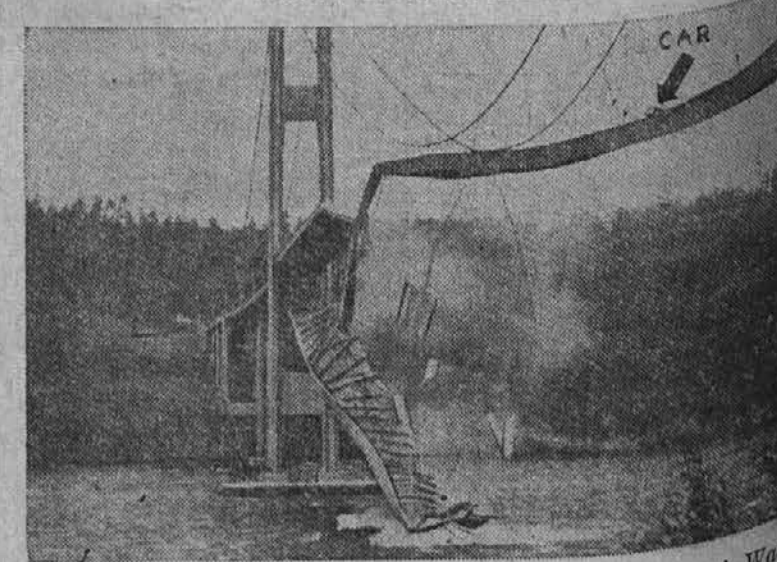
Na sliki vidimo podrtine visečega mostu pri Tacomi, Wash., ki se je te dni podrl, o čemer smo že poročali med dnevnimi novicami v našem časopisu.
