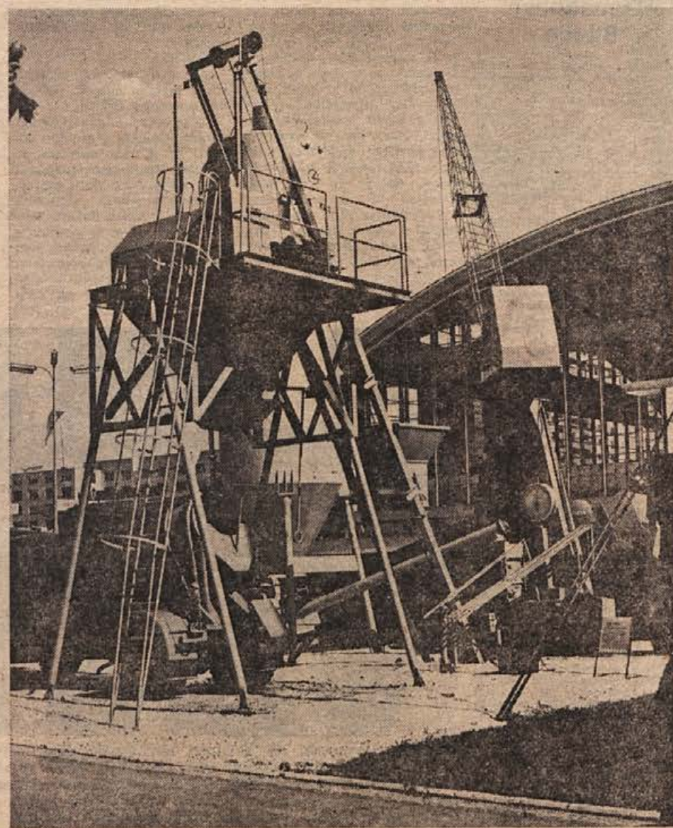
ITASOVA polavtomatska betonarna z zmogljivostjo 15 kubičnih metrov betona na uro
