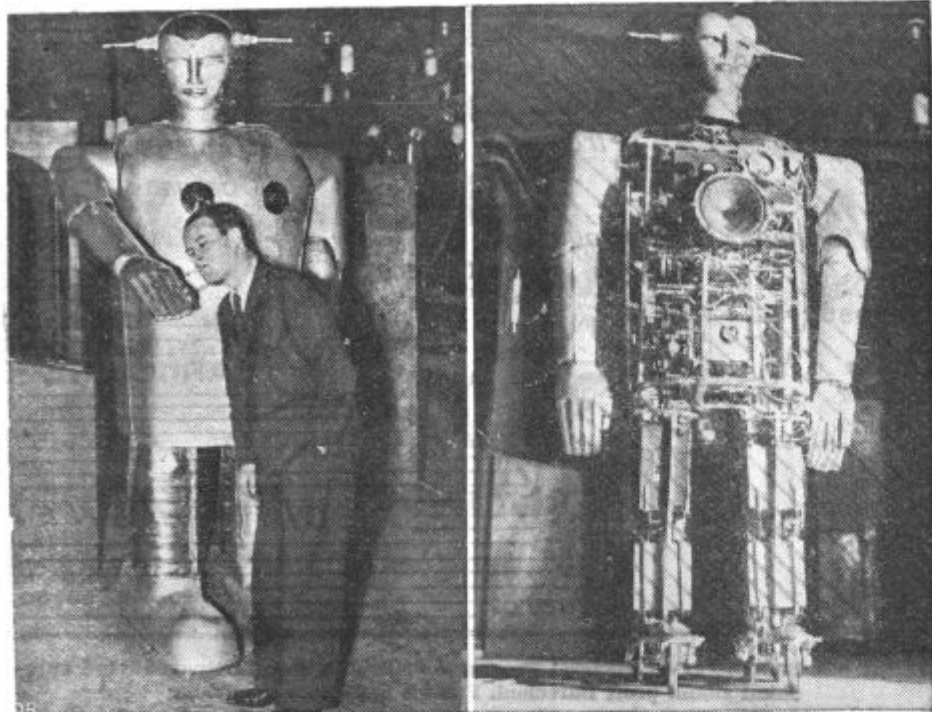
ROBOT »SABOR«. Robot z imenom »Sabor«, ki ga je zgradil Avgust Huber iz Nieder- teuffena pri Appenzellu. Na levi vidimo robota, ki prižiga gospodarju cigareto; na desni vpogled v robotovo notranjost
