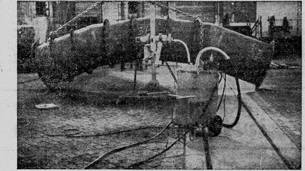
Po večdnevem preizkušanju naprav je bila v nedeljo spuščena v poskusni pogon hidrocentrala Došnica pri Demir-Kapliji. Vsi trije generatorji bodo delovali na električne energije. To je četrta hidrocentrala, ki so jo zgradili v Makedoniji po osvoboditvi. Na sliki: Kontrola varilskih spojev na tlačni cevi za hidrocentralo Došnica v tovarni metalnih konstrukcij »Franc Leskošek« v Mariboru.
