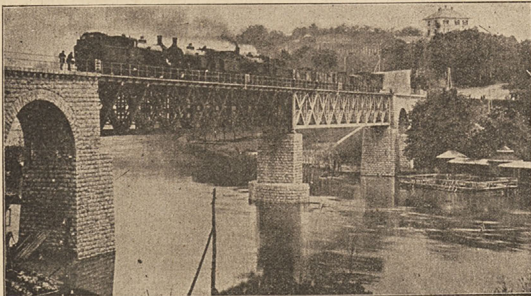
Pred otvoritvijo belokranjske železnice: Obtežilna poskušnja novega mostu čez Krko.
