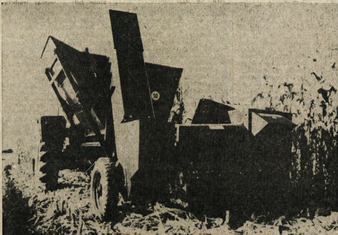
KOMBAJN ZA OBIRANJE KORUZE KK 30. Tehnični podatki: dolžina 4 m, širina 2,75 m, višina 2,4 m, zmogljivost 0,15-0,35 ha/h, potrebna moč 25 KM; LICKALNIK: valji: 3 železni in 3 gumijasti, dolžina valjev 1,13 m, drobilec z 9 noži; BUNKER: zmogljivost 1,5 m 3 , praznjenje hidravlično, višina praznjenja 1,95 m
