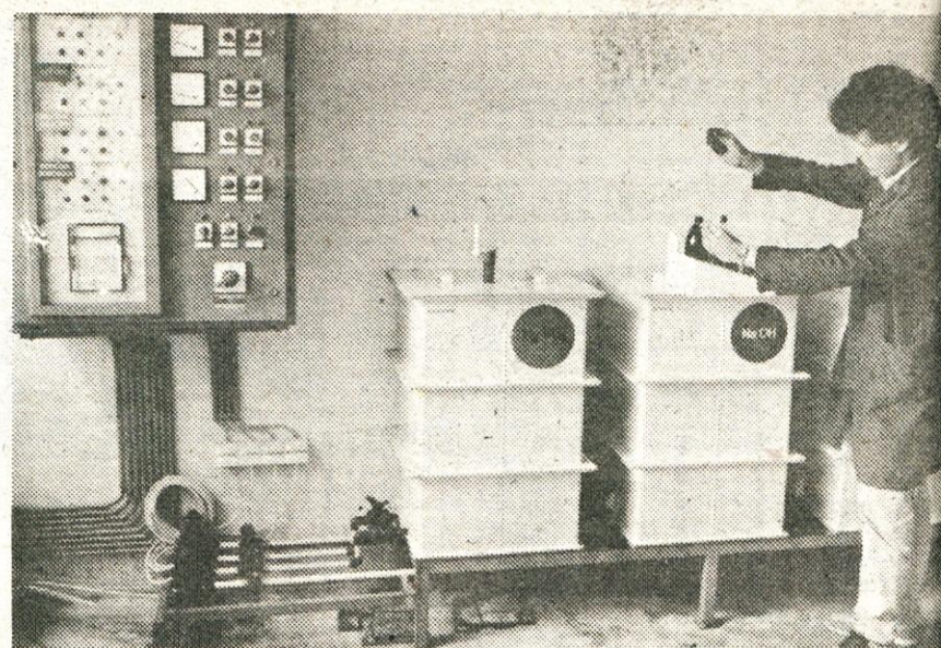
Nova čistilna naprava v Radomljah popolnoma zagotavlja ustrezno kakovost odpadnih voda. Na sliki: delo na Šrajevi čistilni napravi.
