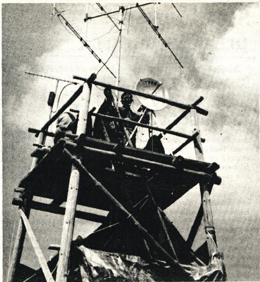
Ob letošnjem tekmovanju za Teslov memorial na visokih frekvenčnih obsegih 432 MHz, 1296 MHz in 10 GHz — člani Radio kluba Domžale.
