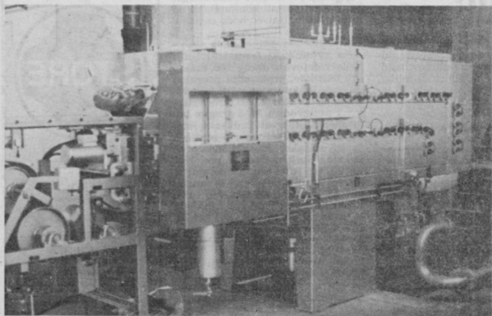
Linijo termične obdelave sestavljajo: pretočna peč z oljno kopeljo, kjer obročke okalijo, da postanejo bolj trdi, peč za popuščanje notranjih napetosti, plinski generator in šestbarvni točkovni registrator za nadzor. Vse to v Žični že imajo, čakajo le še na plinsko postajo.
