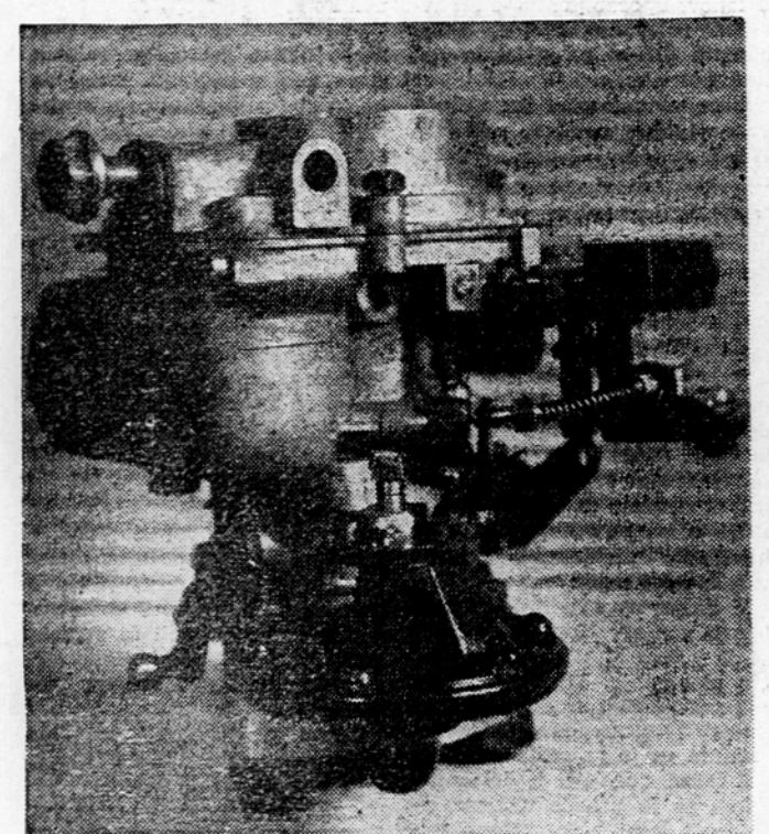
Aparat »Rams«, montiran na razplinjač »Solex«.
