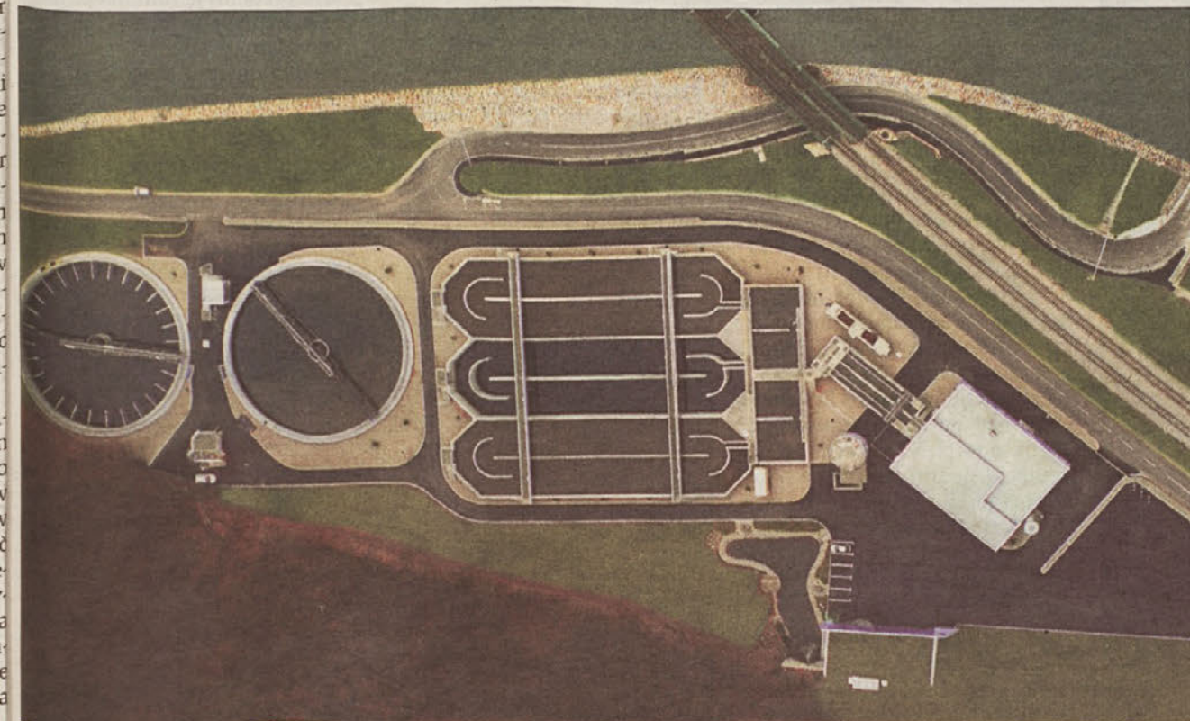
Pogled na celjsko čistilno napravo iz ptičje perspektive
