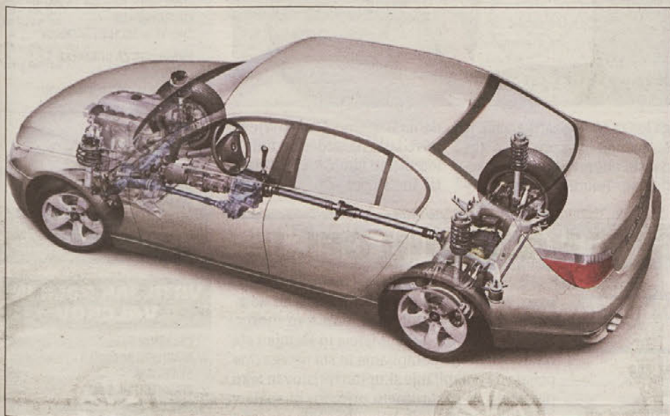
Serijski 5 in štirikolesni pogon
