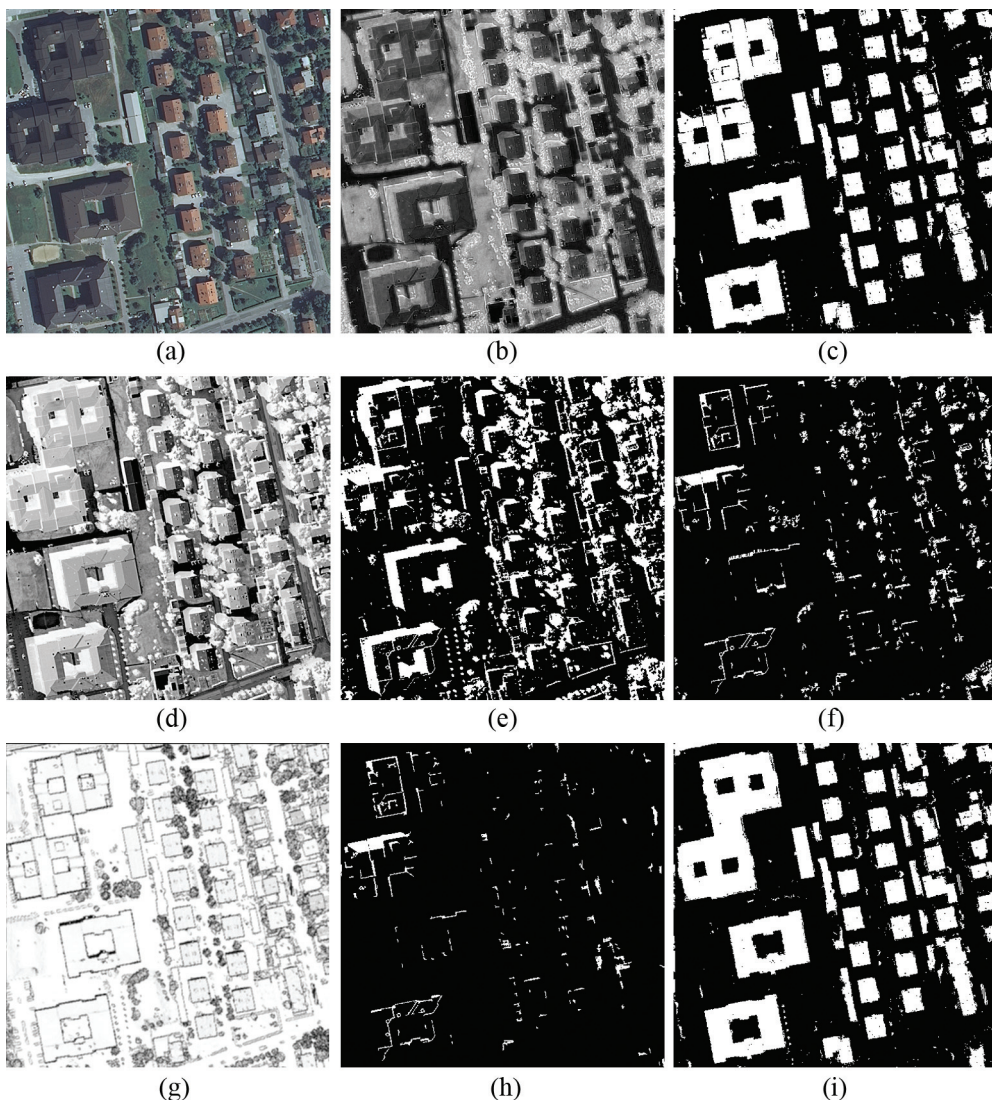
Slika 4: Izdelava začetne maske stavb
