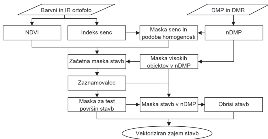
Slika 1: Diagram poteka zajema stavb iz DMP in ortofota
