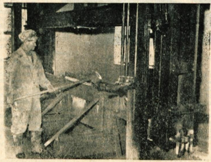
Polnojarmenik ali »gater« za rezanje blokov v plošče
