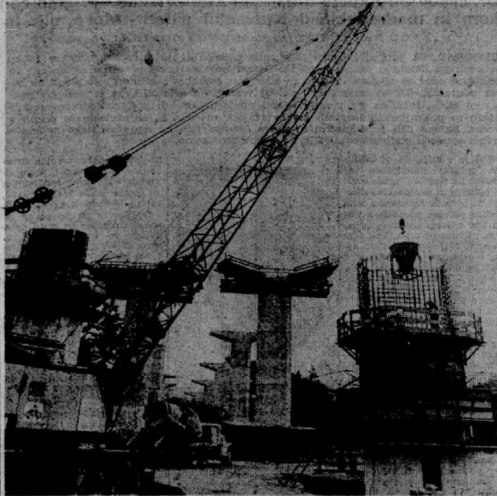
VIADUKT NA RAVBARKOMANDI RASTE - Še pred nekaj meseci so imeli graditelji velikih objektov na hitri cesti Vrhnika-Postojna precejšnjo zamudo, kar velja zlasti za skoraj 600 m dolgi viadukt pri Ravbarkomandi (na sliki). Zdaj pa so s pospešenim delom zamude nadoknadili. Foto: E. Selhaus
