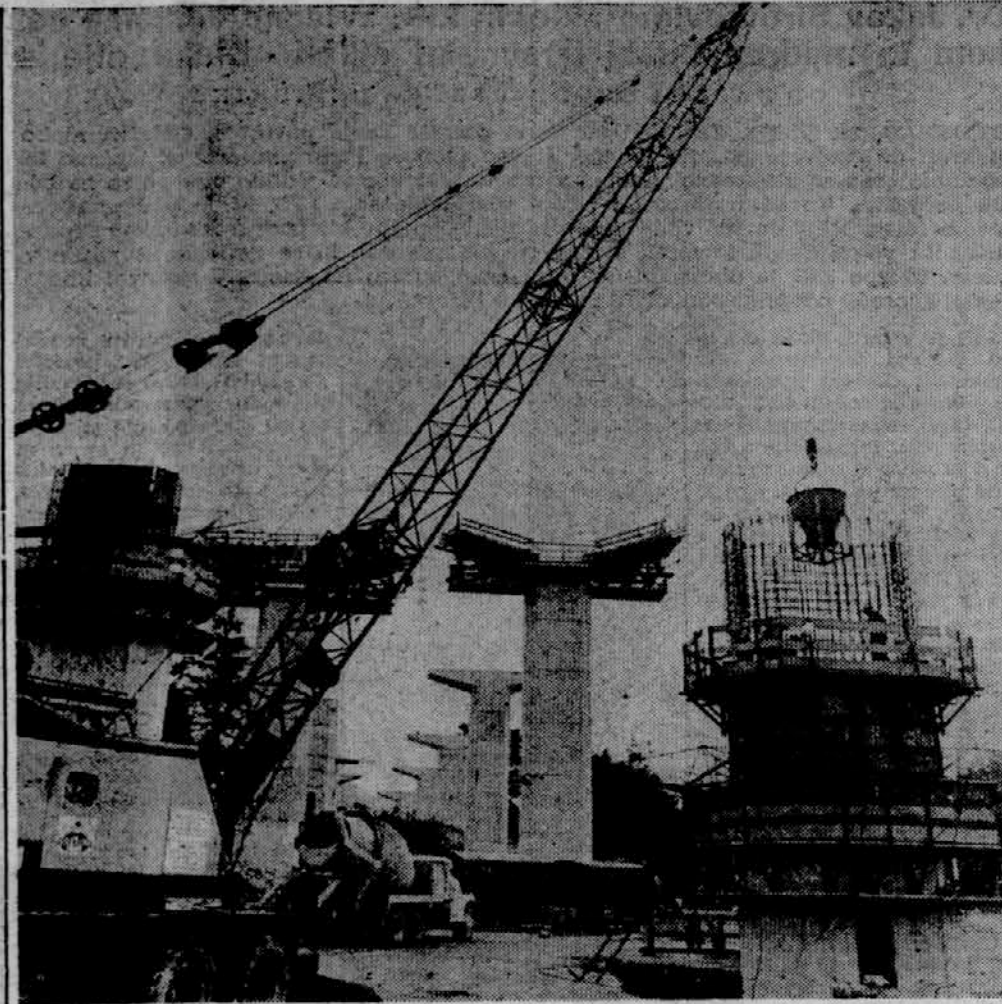
VIADUKT NA RAVBARKOMANDI RASTE — Se pred nekaj meseci so imeli graditelji velikih objektov na hitri cesti Vrhniko-Postojna precejšnjo zamudo, kar velja zlasti za skoraj 600 m dolgi viadukt pri Ravbarkomandi (na sliki). Zdaj pa so s pospešenim delom zamude nadoknadili. Foto: E. Selhaus
