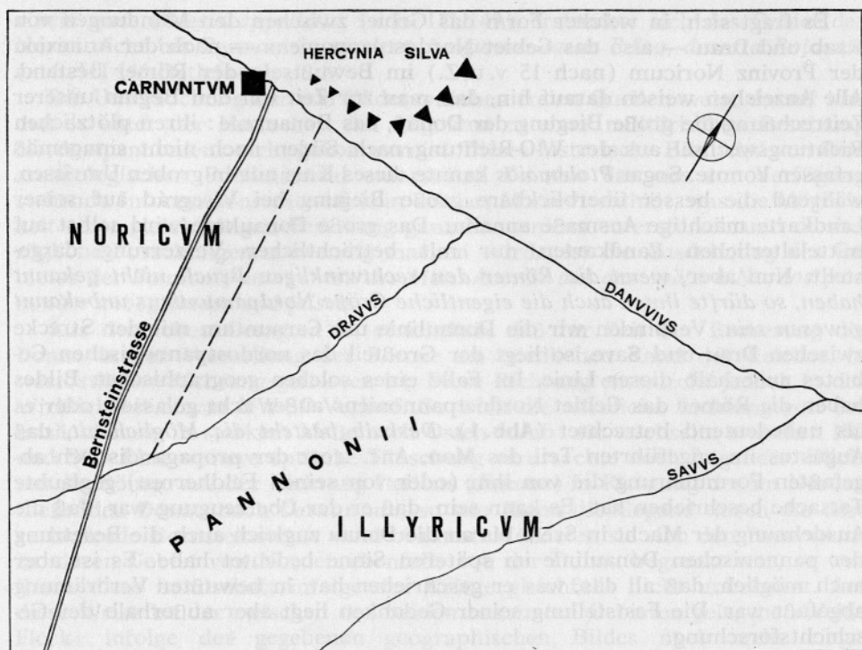
1 Ursprüngliche Vorstellung des Donauverlaufes. Rekonstruktionsversuch. — Prvotna predstava donavskega toka. Rekonstrukcija
