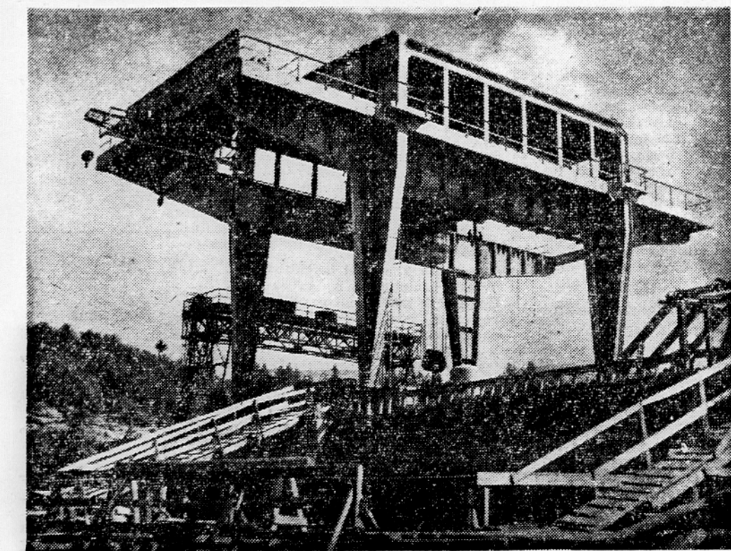
Najnovejši posnetek iz HC Yuzenica: veliki 150 tonski žerjav v obratu
