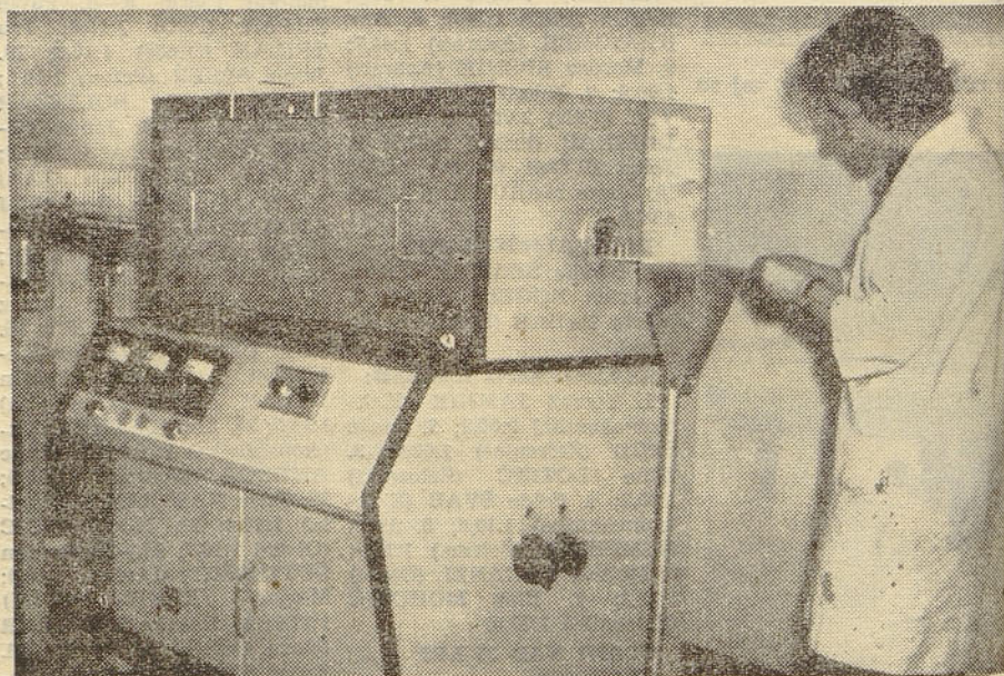
Iz tovarne polprevodnikov: tov. Hilda pri difuziji šilda pri peči
