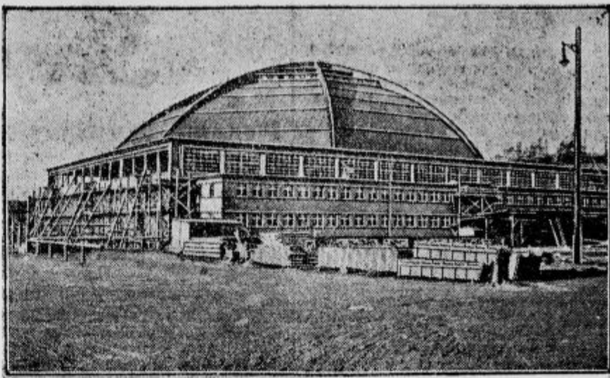
Nova veletržnica v Leipzigu, ki bo največje poslopje v obliki kupole na svetu. Kupola sloni na osmih oporah; ima 67 metrov v premeru in pokriva 6000 kvadratnih metrov ploskve. Poslopje je zgrajeno iz železobetona.
