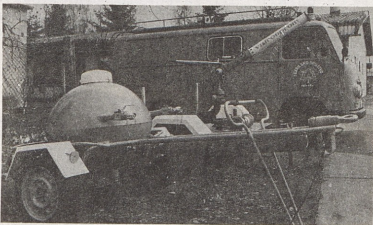
Sodobna gasilska sredstva, s katerimi je opremljeno IGD Agis
