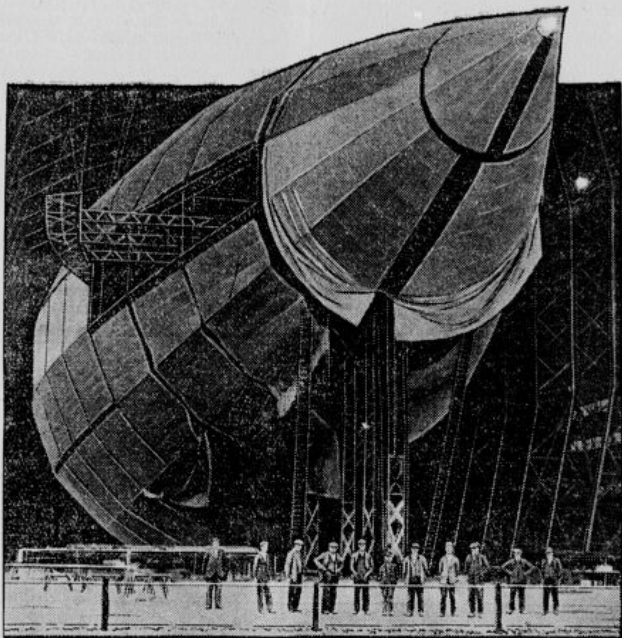
Največji zrakoplov na svetu. V Cardingtonu An. leži že več mesecev gradijo orjaški zrakoplov R 100, čigar motorji bodo imeli 4000 konjskih sil.
