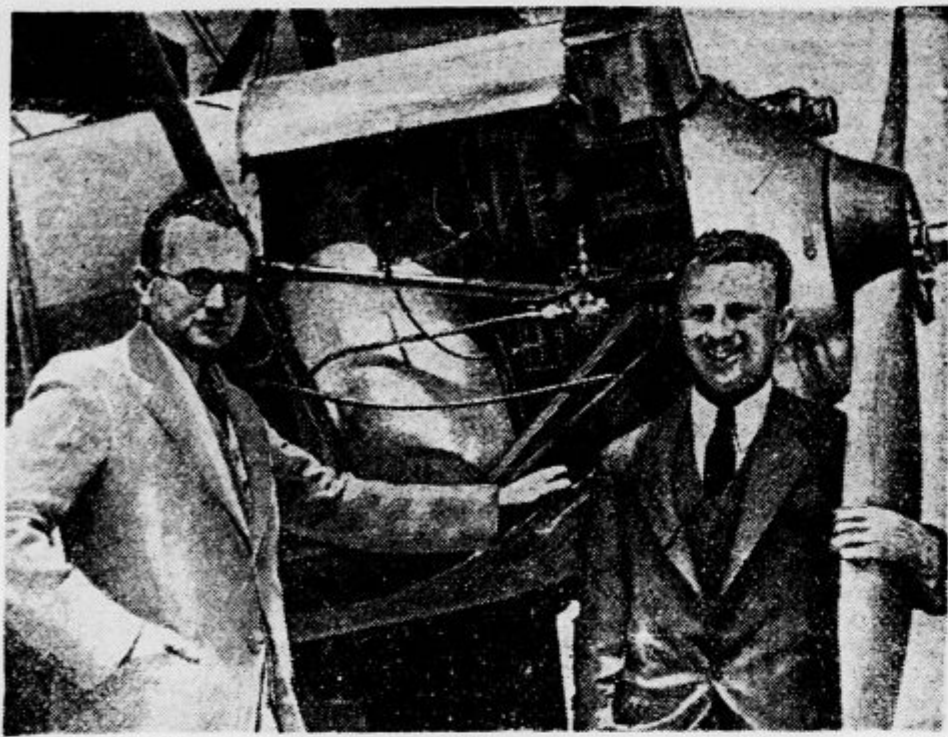
▼ Oaklandu (Kalifornija) sta brata William in George Besler zgradila letalo, ki ga žene stroj na paro. Dosedanji poleti so dobro uspeli
