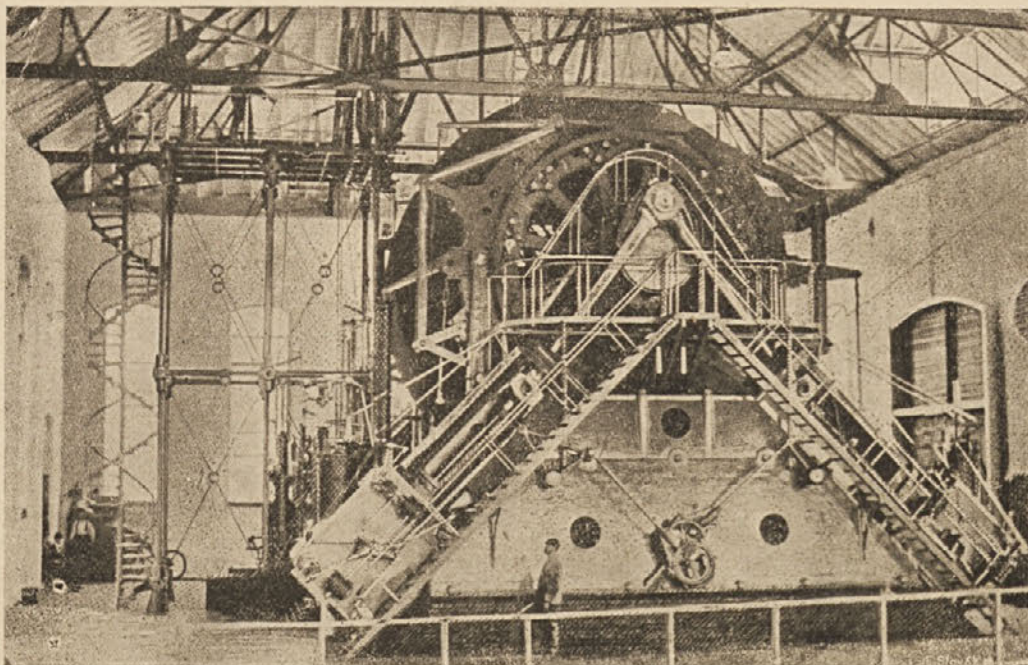
Največji stroj na svetu za vzdigovanje rude.
