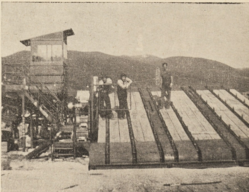
Delavci iz DO IMD — TOZD SIMD in TOZD EIMD so izvajali dela pri postavitvi nove žage in transporterjev gozdnega gospodarstva Delnice, na Hrvaškem.
