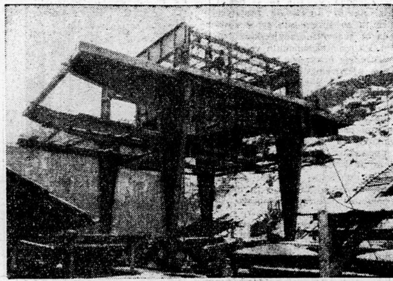
Na gradbišču hidrocentrale Moste lepo napredujejo montažna dela. Velika zapornica na območnem rovu je že v obratu. V dovodnem tlačnem rovu, po katerem bo odtekala voda iz umetnega jezera do centrale, sedaj montirajo delavci »hidromontaže« glavno in pomožno zapornico. Nad strojno centralo, ki je zgrajena na obrežju Save globoko pod zemljo, so nedavno postavili velik portalni žerjav za montažo in poznejši remont turbin in generatorjev. Ta žerjav, ki ga vidimo na sliki (tik pred dovršitvijo) že služi svojemu namenu, namreč montaži prvega turboagregata.
