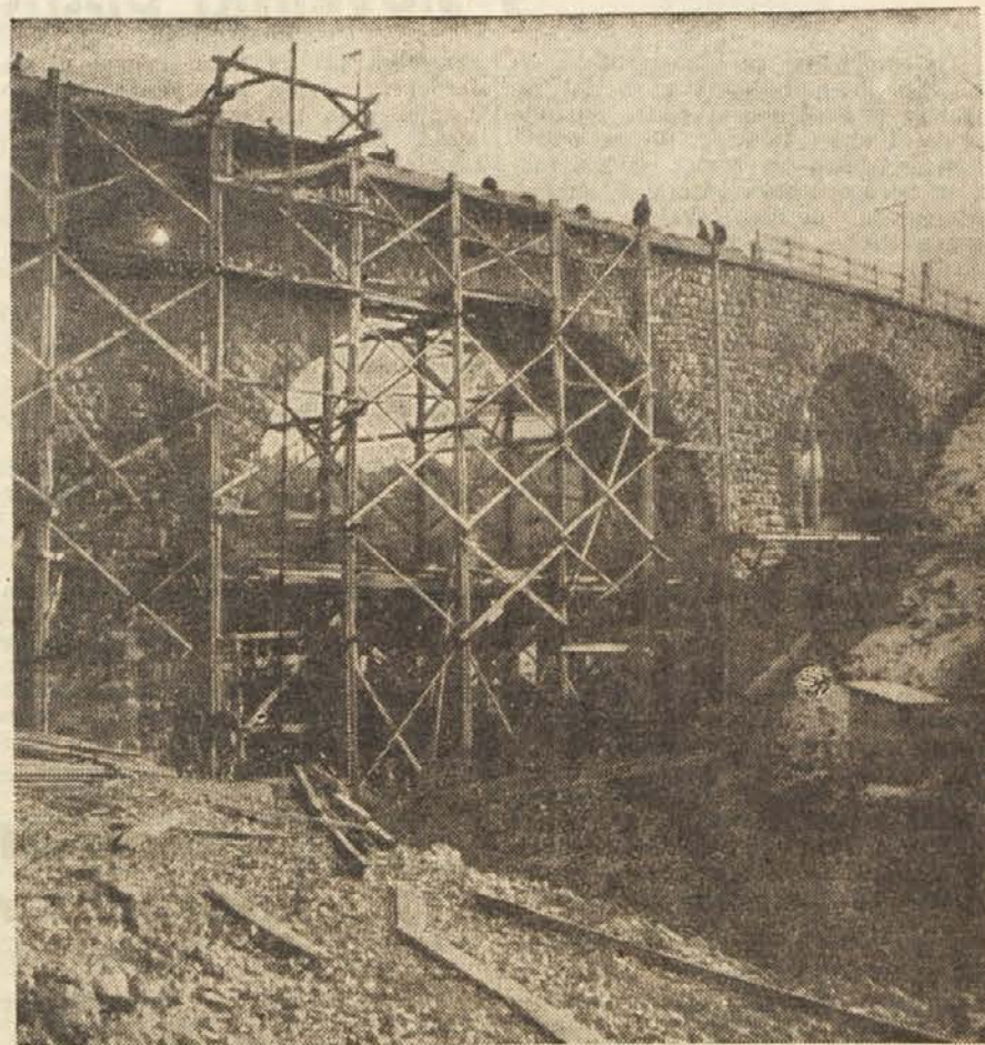
Obnovljeni železniški most čez Krupo je dolg 86 m. Za obnovitev je bilo potrošenih 125 vagonov gramoza, 18 vagonov cementa in pet ton železa. Pred začetkom obnove je bilo treba razrušiti 322 m 2 starega viadukta, izkopati nove temelje in napraviti 745 m 2 opaža za konstrukcije. Dalje je bilo treba narediti 1044 m 2 betonskih del, 255 m 2 kamenite obloge in 450 m 2 svinečne izolacije, iste, kakršna je položena na obojskem viaduktu. Posebno pohvalo pri gradnji mostu zasluži tesarški mojster Sušteršič Ignac in železniški nadzorniški pripravnik Besednjak Boštjan. Mnogo truda pa je v delo vložila tudi vsa okoliška mladina in so se posebno izkazale pri delu mladinke iz vasi Gribelj in Krasinca.
