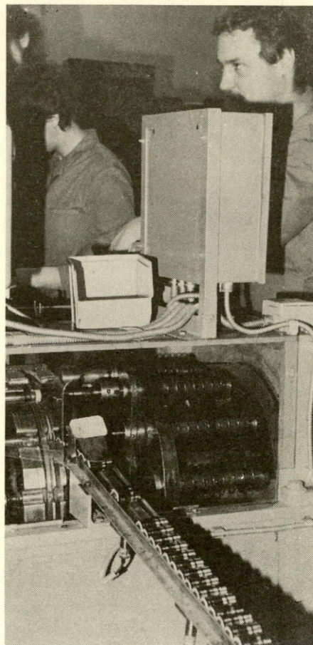
Tik pred robljenjem oziroma zapiranjem baterijskega člena v kovinski plašč
