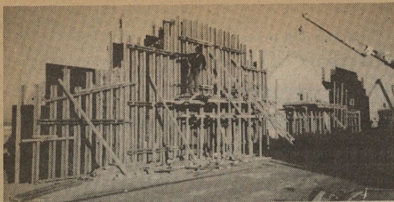
Betonsko zidovje smo opažili po tamkaj domačem sistemu DOKA. Delo je opravila skupina tesarjev iz GE Jesenice ob pomoči delavcev iz Egipta.
