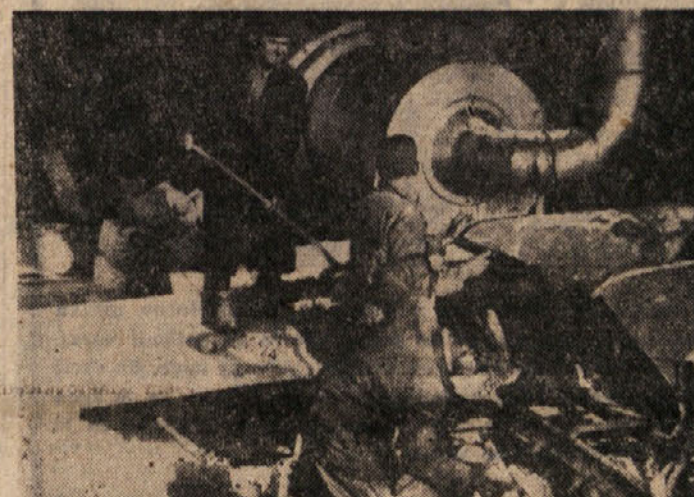
To je rotacijska peč na obratu Mokro polje. Nadomestila je prejšnje enostavne zidane peči. Z lopatami nametajo v odprtino vlažen pesek, na drugem koncu peči pa se že siplje suh v vrečo
