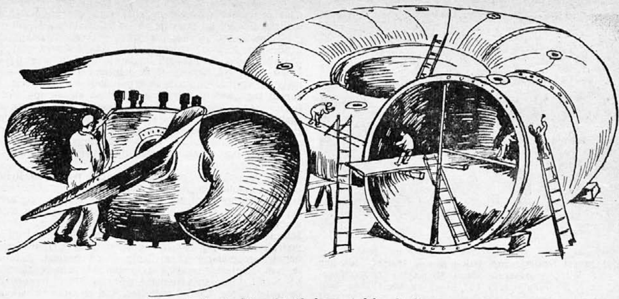
Vodne turbine, ki jih bomo izdelovali doma
