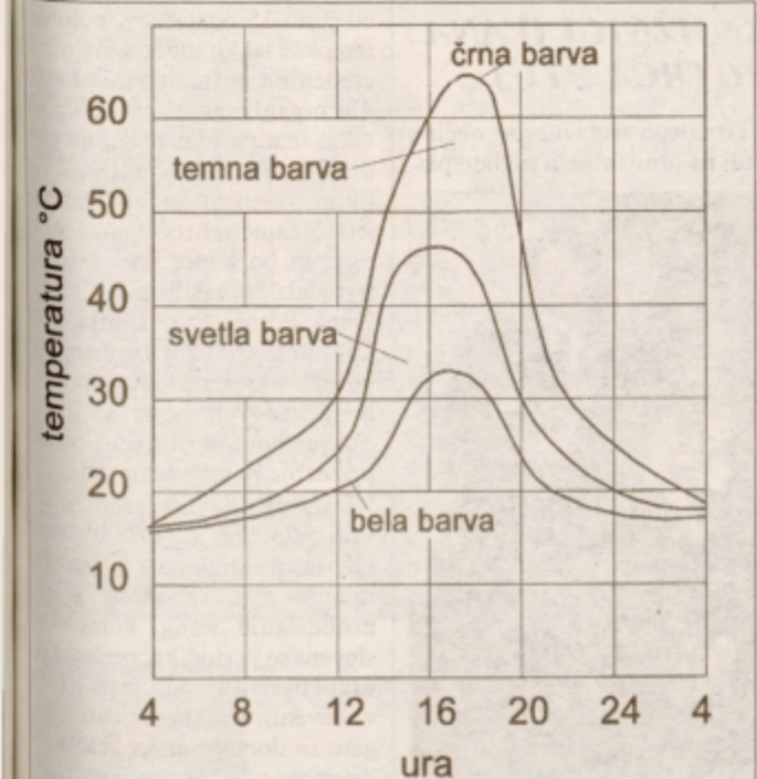
Vpliv barve zunanega ometa na površinsko temperaturo konstrukcije
