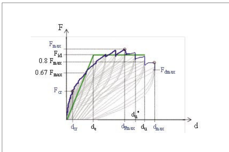
Slika 14 • Bilinearna idealizacija histerezne ovojnice po kriteriju 2/3 F_{max}
