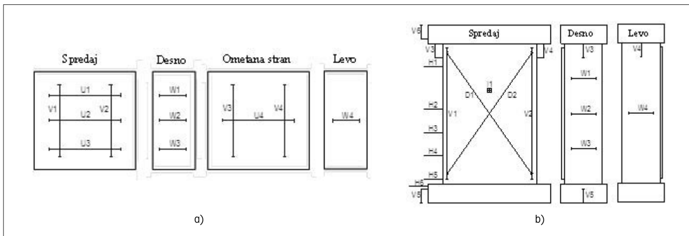
Slika 8 • Postavitve merilnih mest pri a) tlačnih preizkusih in b) strižnih preizkusih
