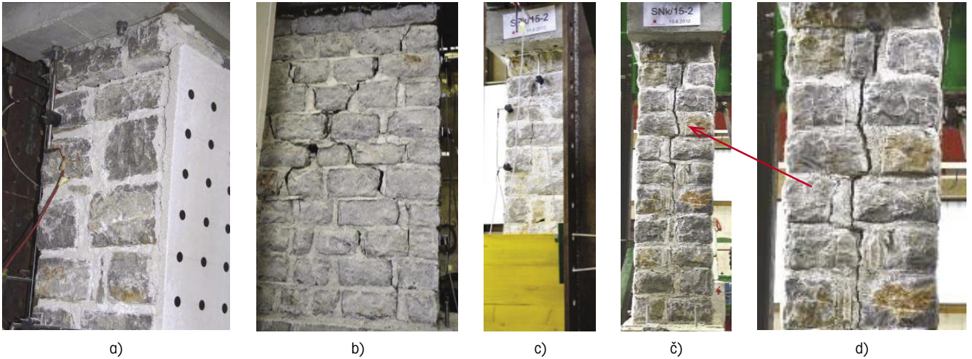
Slika 11 • a) Upogibni mehanizem z odpiranjem maltno spojnice med prvima vrstama kamnitih blokov pri testu 2 – SNk-7,5-1, b) diagonalne strižne poškodbe zidu po testu 13 – SPk-15-2 ter c) razpoka med slojema po istem testu, č, d) razpoka med slojema zidu po testu 14 – SNk-15-2
