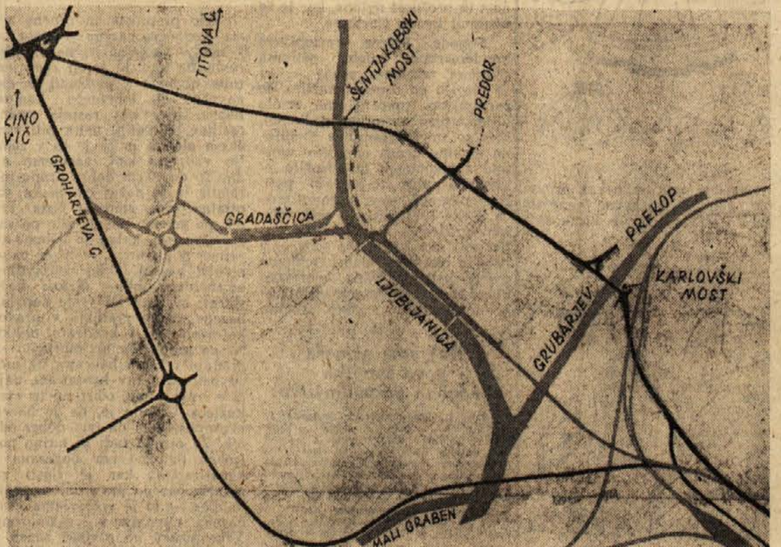
Debelo tiskani črti predstavljata trase vpadnice po I. varianti (zgoraj) in po III. varianti (spodaj). V sredi je trasa po II. varianti; črtikani del pomeni cesto v prvi etapi variante
