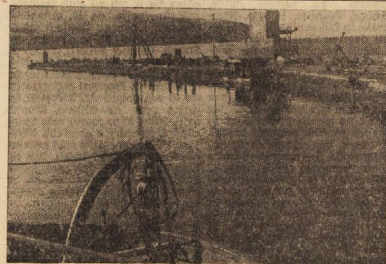
Koper: obnova lukobrana v starem pristanišču
