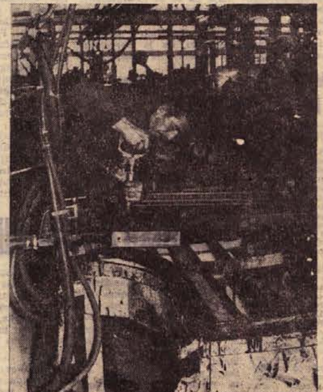
Točkovno varjenje sprednjih vrat vozila IMV
