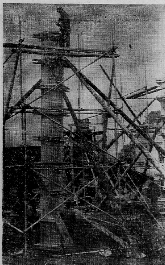
Dela na novem objektu pri Dolgem mostu na Viču, ki bo obenem most čez Mali graben in nadvoz nad železnico, so zaradi slabega vremena začasno prekinjena. Novi most, ki so ga projektirali pri »Projektu« - nizke zgradbe, so pričeli graditi decembra 1989. Pri podjetju »Slovenija ceste«, ki izvaja gradbeno dela, so menja, da bo novi objekt končan v prvi polovici tega leta Foto: Z. Deniša
