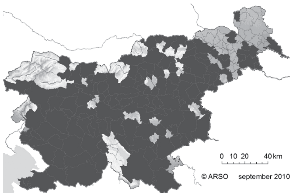
Občine (temno), kjer so bile zaradi obilnega septembrskega deževja potrebne intervencije, med njimi je seveda tudi trzinska (Vir: Izjemno obilne padavine od 16. do 19. septembra 2010, spletne strani ARSO).
