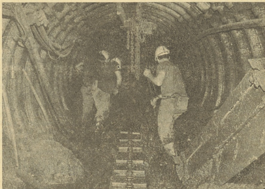
Dne 24. maja t.l. sta vdor vode in vdor blata povzročila v Terezija II polje, kota 170 v jami Ojstro, veliko škodo. O tem smo v prejšnji številki glasila že obsežneje pisali. Dela pri čiščenju proge oziroma kota dobro napredujejo. (Foto J. Kirič)
