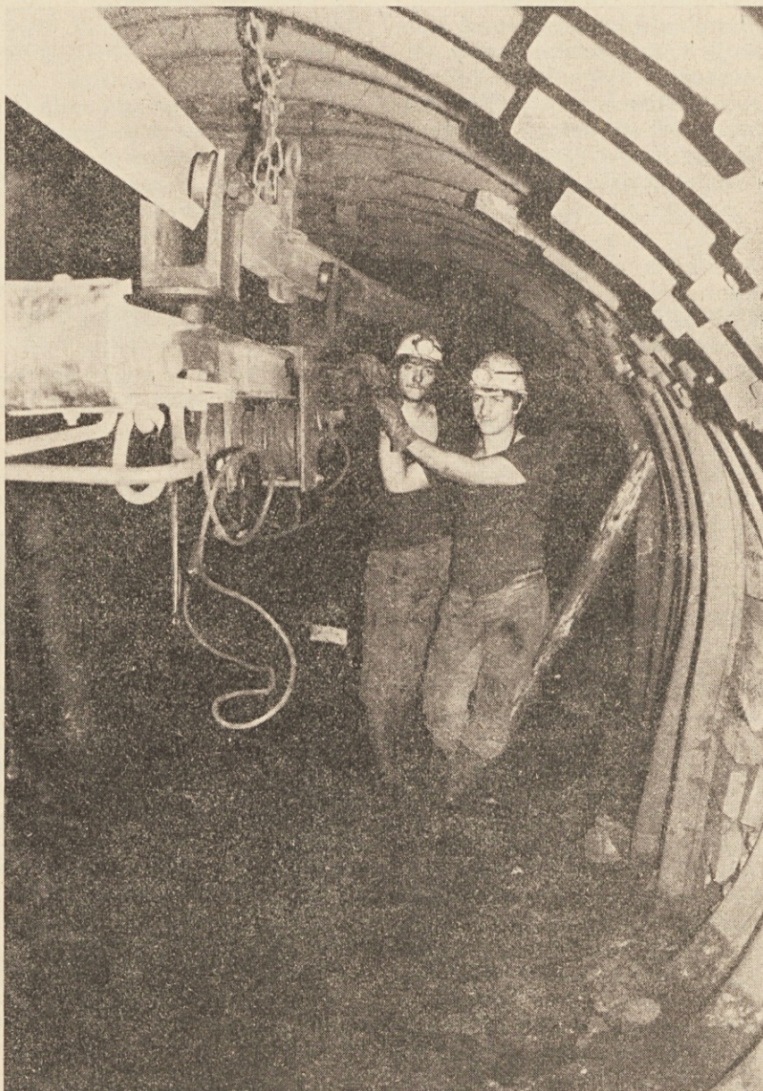
Rudarja Mesud Rabihič in Miloš Točakarič pri spravilu materiala z visečo žičnico — monorail, na koti 160 v jami Ojstro.
