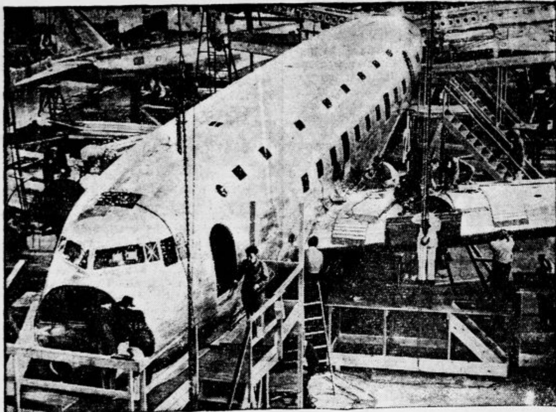
V ladjedelnici Douglas v Santi Monici izdelujejo letalo, ki bo vzdržalo tudi največji pritisk pri poletih v stratosfero. V gondoli bo prostora za 42 oseb, aeroplan bo imel 4 motorje in bo letel z brzino 350 km na uro
