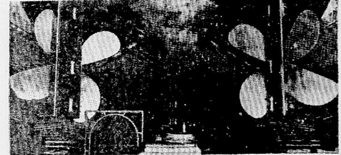
Pred kratkim so končali s preizkušanjem ogromnih propelerjev iz litine nitida, aluminija in bronca. Ladja »Punta Cabrian« je celo leto plula s propelerjema, od katerih je bil eden iz nove litine, drugi pa iz jekla. — Na sliki vidimo obo propelerja po enem letu: jekleni propeler na levi je precej poškodovan zaradi lesa in drugih stvari, v katere se je med vožnjo zadel, desni, ki je iz nove litine, pa je takšen, kot bi bil nov.
