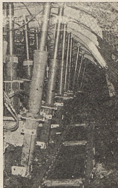
Pogled na zadnji del mehaniziranega širokega čela s samohodnim podporjem Marrel-Hydro — z bananami
