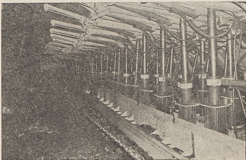
Pogled na prednji del mehaniziranega širokega čela v Zg. VII. polju jame Trbovlje, s samohodnim hidravličnim podporjem Marrel-Hydro
