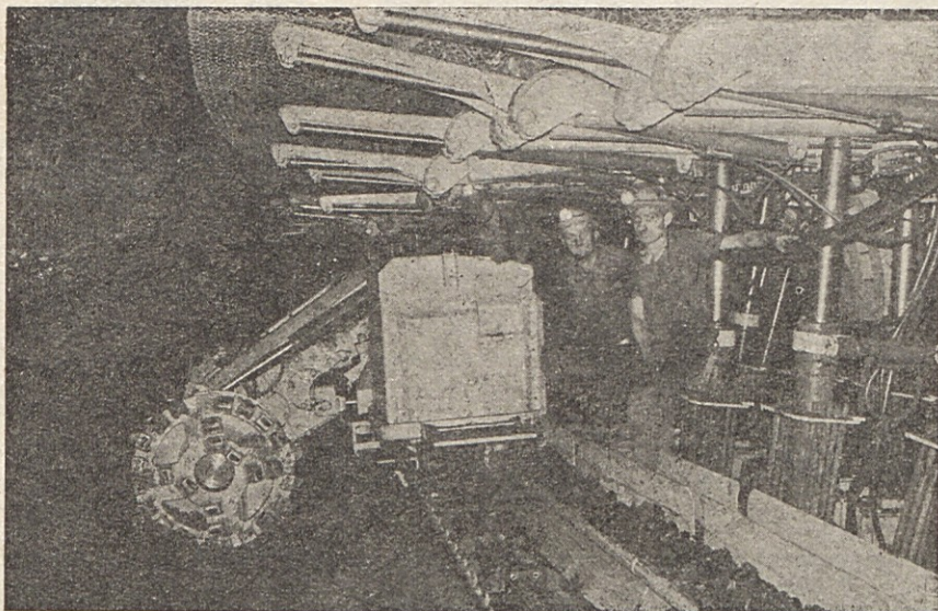
Pridobivalni stroj Revageuse z upravljači tega stroja, pri priučevanju na čelu Zg. VII. polja jame rudnika Trbovlje
