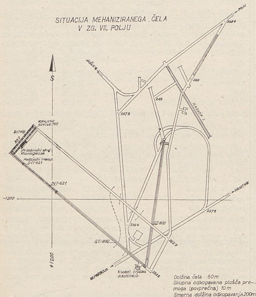
Skica: Situacija mehaniziranega čela v Zg. VII. polju jame TOZD rudnik Trbovlje
