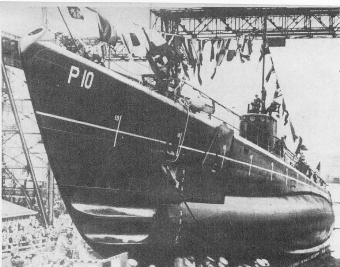
Na levi: Sprednji del podmornice gleda proti bregu, zadnji del pa se prvi skriva pod vodo Spodaj: Sprednji del podmornice razločno kaže 4 odprtine, skozi katere bodo streljali torpede.
