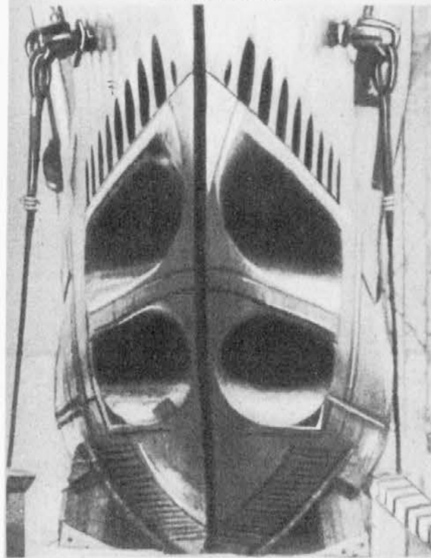
Na levi: Sprednji del podmornice gleda proti bregu, zadnji del pa se prvi skriva pod vodo Spodaj: Sprednji del podmornice razločno kaže 4 odprtine, skozi katere bodo streljali torpede.
