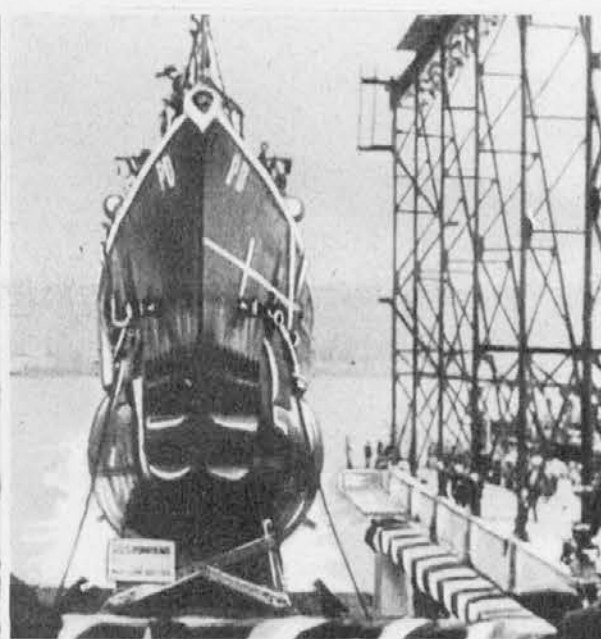
Spodaj: Najbolj nevaren je trenutek, ko je ladja na pol v vodi, na pol na suhem. Če pre- stane to nevarnost, potem mirno zaplava po morju.
