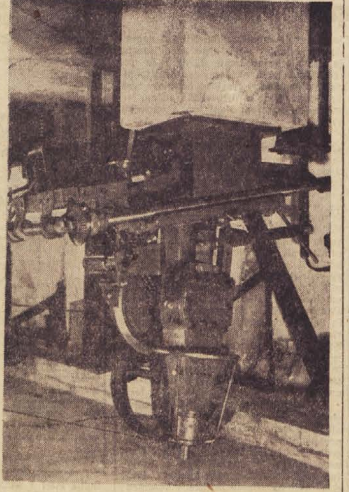
Doma izdelani nasekavalni stroj za nasekavanje pil. Napravili so tri take stroje
