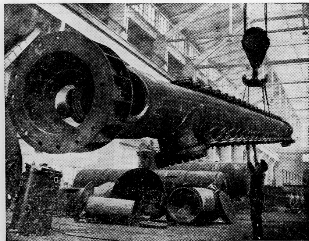
Na sliki vidimo izdelovanje opreme za degazolnažo v Dolnji Lendavi. Opreme za degazolnažo izdelujejo v Ameriki, Angliji in Nemčiji. Opremo za Doljno Lendavo pa izdeluje prvič domača Tovarna parnih kotlov v Zagrebu. Opremo je projektiral inž. Terzić iz Instituta za nafto. Strokovnjaki menijo, da bomo prihranili samo pri izdatkih, ki bi sicer šli tujim tovarnam, okrog 200 milijonov dinarjev. Največja vrednost našega izdelka pa je v tem, ker bomo v naših naftnih pralah pospešili predelavo plina in bodo tako prihranki še veliko večji. Kakor je znano, so v degazolnaži predeluje zemeljski plin v razne spojine in se tako mnogo koristnejše izkorišča, kakor če bi se uporabljal neposredno kot pogonsko sredstvo ali kot gorivo. Skupno bo tovarna izdelala za Doljno Lendavo 6 takih kolon, kakršne goraj del vidimo na sliki.
