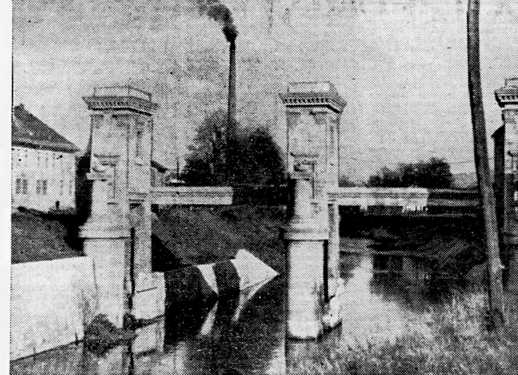
Nova zatvornica na Ljubljanci dlk pred Cukrarno je bila zgrajena že pred vojno, vendar je tedaj niso več utegnili popolnoma opremiti. Mestni občinski odbor Ljubljane je letos naročil vso manjkajočo železno opremo v tovarni »Franc Leskošek« v Mariboru in bo zanjo plačal okoli 40 milijonov din. Ko bodo te naprave montirali, bo zatvornica lahko prevzela svojo funkcijo regulatorja vodostaja na Ljubljanci in s tem tudi na Barju. Tedaj bodo lahko odpravili tudi jez na Spici, ki je doslej mnogokrat koristil, pogosto pa je tudi škodoval.
