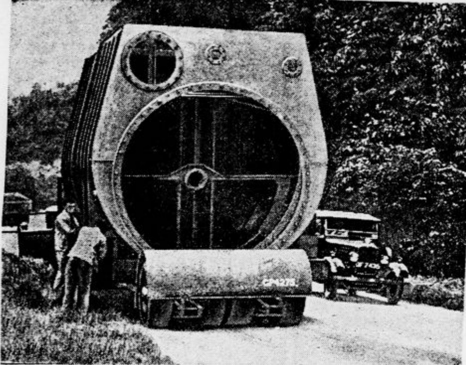
To sliko so napravili v okolici Londona in predstavlja prevoz ogromnega ladijskega kotla, ki tehta 30 ton. Da ne bi oviral cestnega prometa, se je transport vršil ponoči
