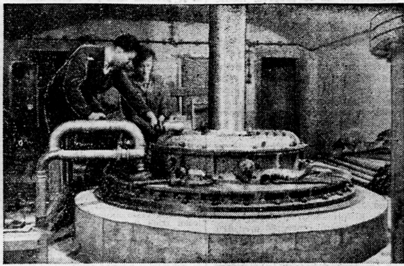
Prva turbina hidrocentrale Moste je že montirana. Na sliki vidimo poslednja dela na vrhu turbine, kjer je ležaj turbine gredil in je priključena regulacijska naprava. Na pokončno gred, ki jo vidimo na sliki, sedaj montirajo generator.
