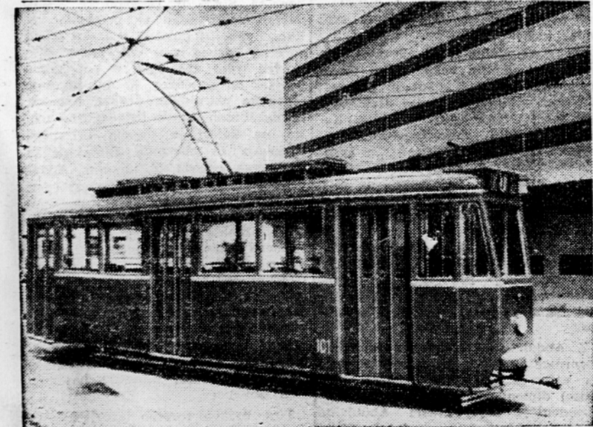
V delavnici zagrebske cestne železnice so izdelali po lastnih načrtih moderen tramvajski voz, ki ga sedaj preizkušajo. Vsi deli voza so doma konstruirani in izdelani. Pogonski motor ima 60 konjskih moči in daje vozilu hitrost do 36 km na uro. Sprejmlja, zadržaja in srednja vrata se odpirajo in zapirajo pnevmatično. Motorje za nove tramvajске vozove bo izdelovala tovarna »Rade Končar« po načrtih konstruktorja inž. Mandla. Tovarna »Rade Končar« bo v bodoče lahko dobavljala take motorje tudi Ljubljani, Beču in drugim mestom.
