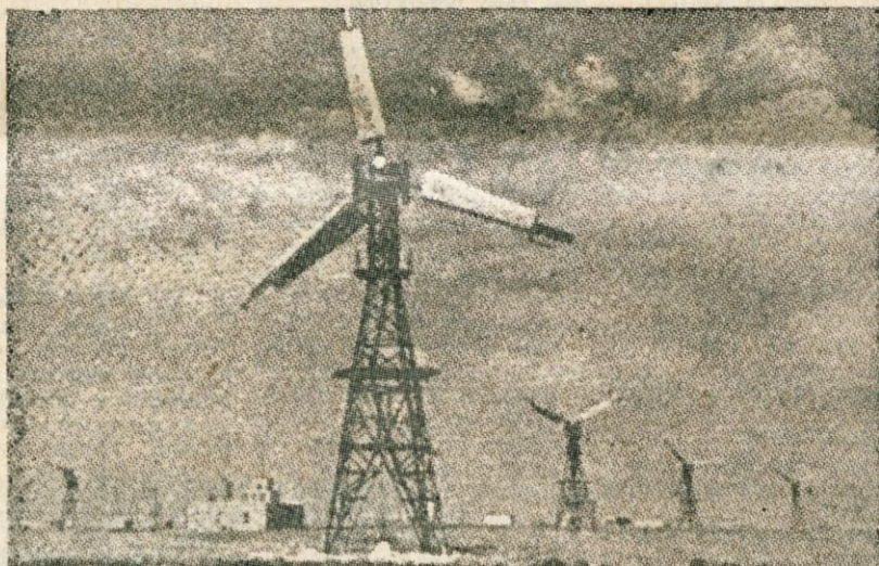
Mlini na veter? Ne, marveč električna centrala v kazakstanski vasi Nova Išimka. Dvanajst vetrnjač poganja ustrezne turbine in agregate. — Praviijo, da ima vas vedno dovolj elektrike zase in za vso sosesčino.
