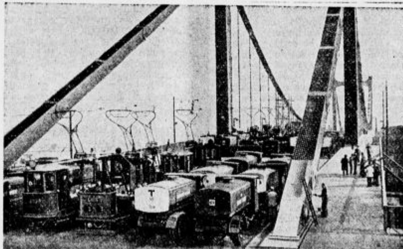
Most dela maturo. — Nedavno so dogotovili most čez Donavo in so ga morali obtežiti s tramvajem, avtomobili in drugimi vozili, da so preizkusili, ali more most vzdržati breme 1.304.000 kg. Most je maturo napravil z odličnim uspehom
