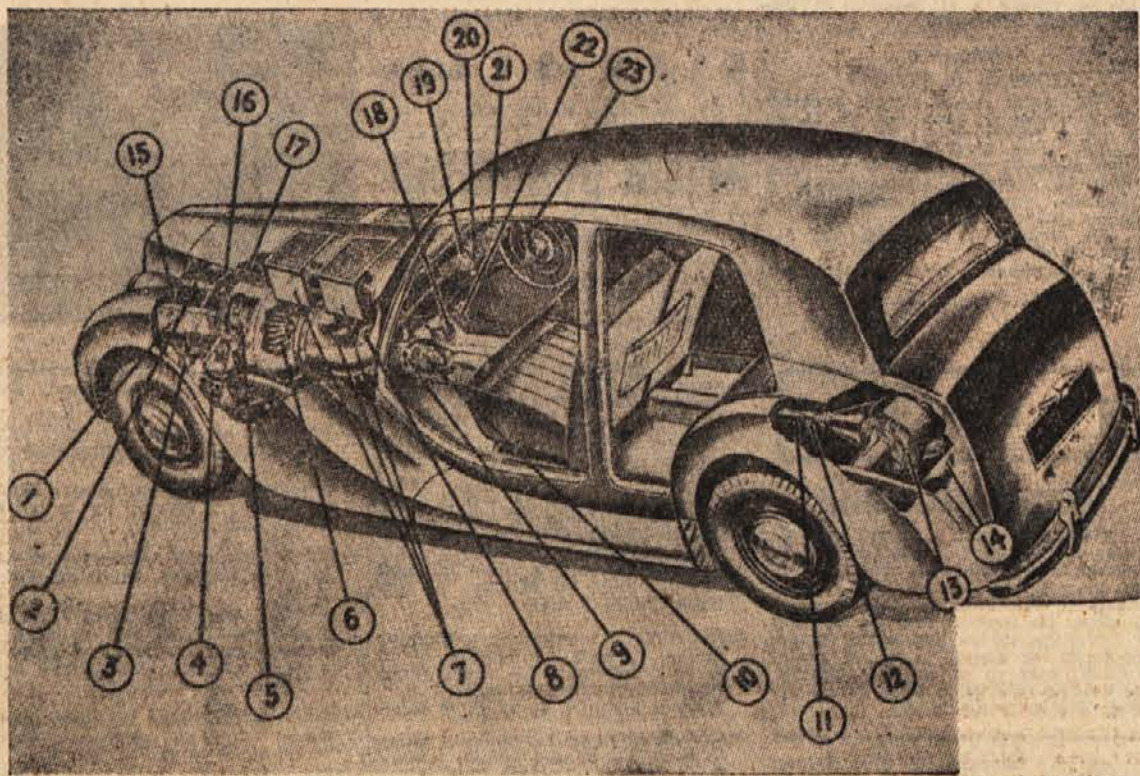
1. Pomožni zaganjač in zračno ustje. 2. Generator. 3. Crpalka — »ventilator«. 3. Neodvisni sprednji prekinjač. 5. Vplinjač. 6. Druga turbina in vplinjač. 7. Predgrejna komora. 8. Reduktor. 9. Obračalnik. 10. Izpušnik. 11. Gonilna os. 12. Univerzalna sklopka. 13. Normalni diferencial. 14. Polnilni tank. 15. Oljni hladilnik. 16. Zaganjač. 17. Lopatice »mlina«. 18. Zavora. 19. Merilec zaloge goriva. 20. Menjalnik za vožnjo naprej in nazaj. 21. Brzinomer. 22. Dovajalec plina. 23. Kazalec smeri.
